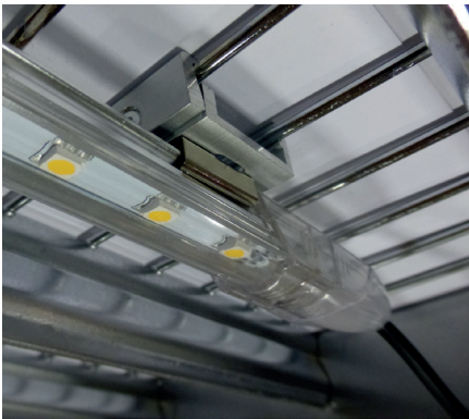
Montage de la LED FOOD en sous face des grilles FL avec le clip monté sur pince.
